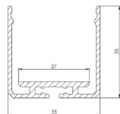
SCALE 1 : 1
